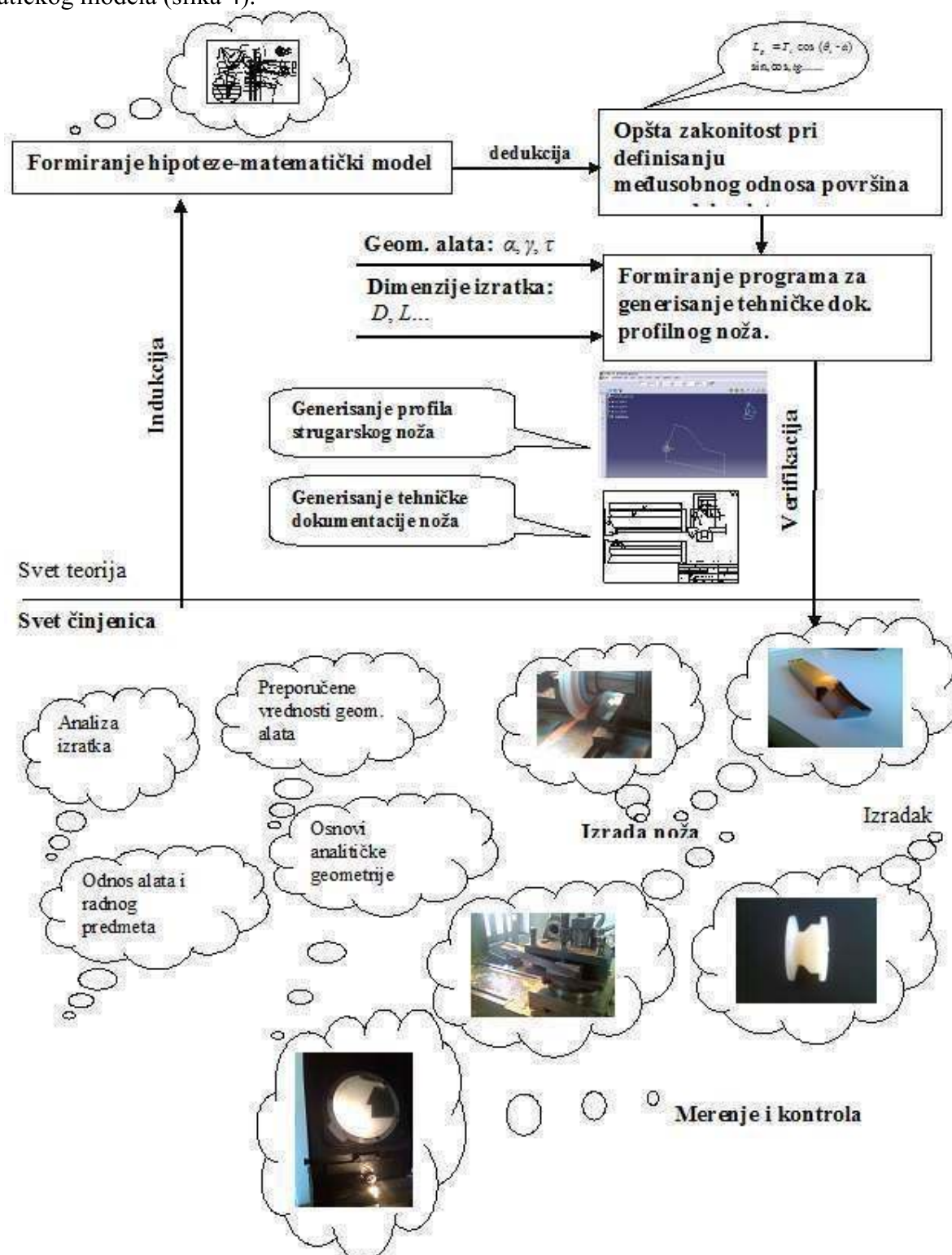
Slika 4. Šematski prikaz metodologije projektovanja prizmatičnog profilnog strugarskog noža
