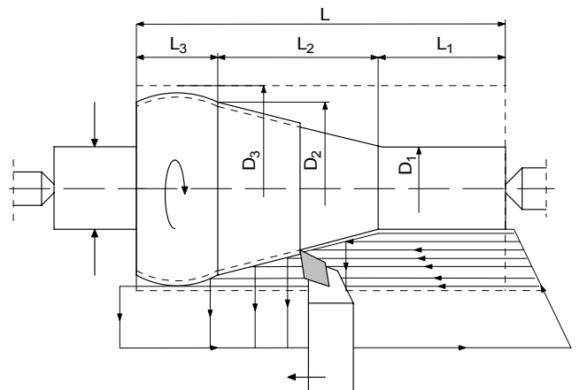
Сложени захват (1 алат за више узастопних површина)
