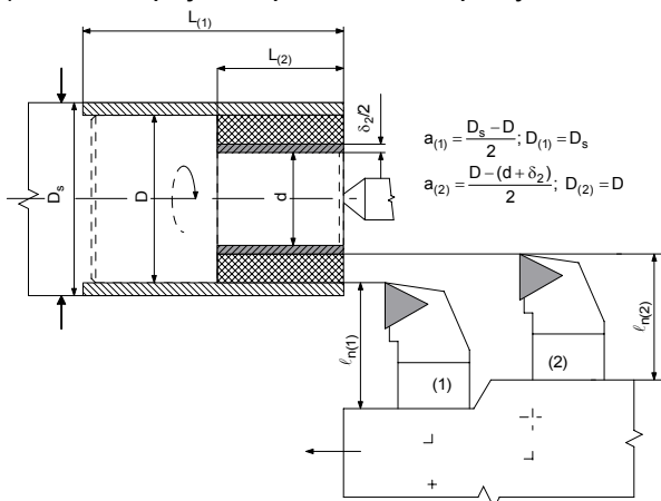
Групни захват (великосеријска производња, робусне машине)
