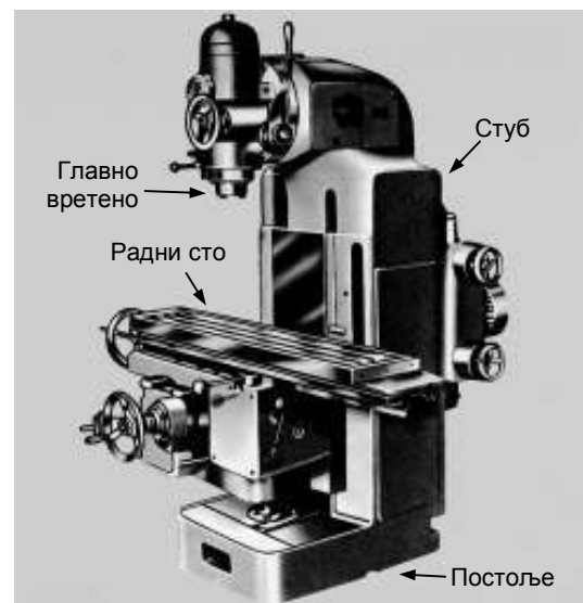
Вертикална глодалица
