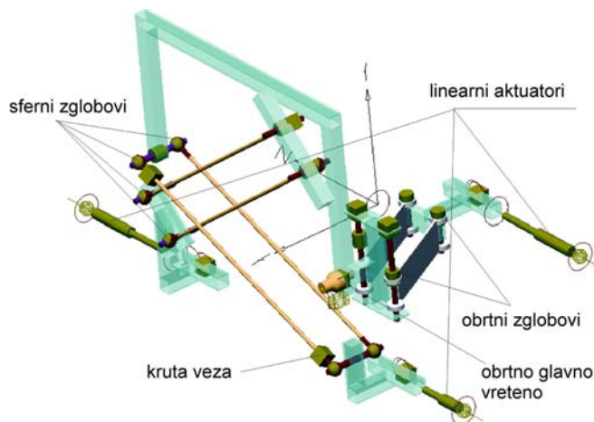
Sl.3 Model za simulaciju troosne paralelne mašine
