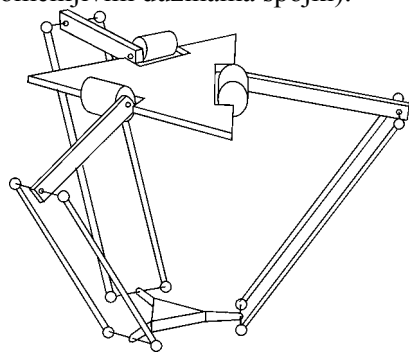
c) MPK sa obrtnim spojkama
