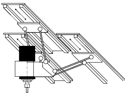
b) MPK sa konstantnim dužinama nogu
